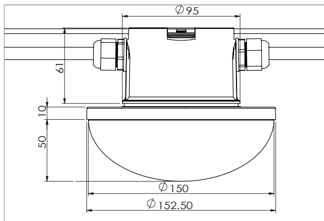
Pendant mounting
